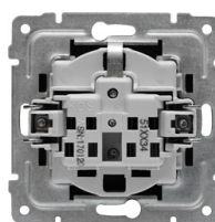
GNIAZDO, widok na kostkę kostka posiada zaciski śrubowe z nakrętką, która nie wypada
