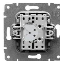
ŁĄCZNIK Z PODŚWIETLENIEM, widok na kostkę, każdy mechanizm można podświetlić elementem neonowym
