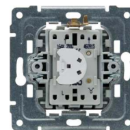
ŁĄCZNIK Z PODŚWIETLIENIEM, widok na kostkę, każdy mechanizm można podświetlić elementem neonowym
